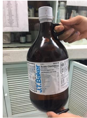
Acido Clorhídrico
