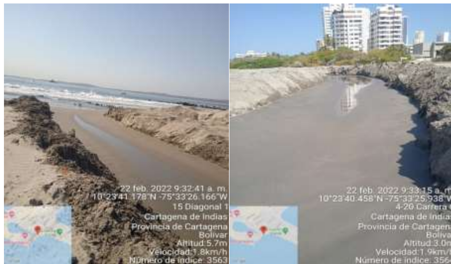
Ilustración 11. Evidencia fotográfica de la obstrucción y/o alta sedimentación en la comunicación natural del Laguito con el mar.
