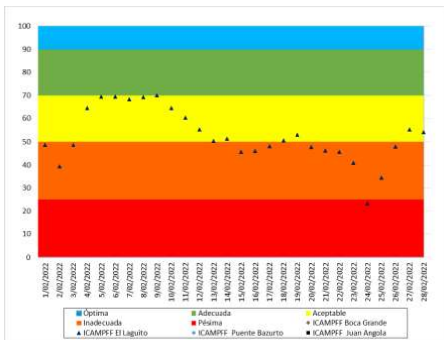
Ilustración 10. Evolución del ICAM pff de la estación del Laguito basado en las mediciones diarias de OD y pH (Confianza del resultado 28%)
