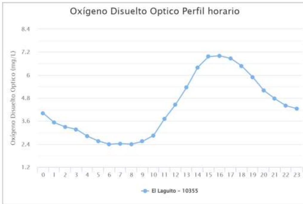
Ilustración 6. Perfil horario de Oxígeno Disuelto Junio estación AG4-El Laguito Fuente: Estudio Actual
