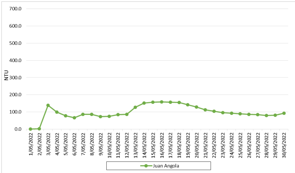
Ilustración 17 Turbidez del agua marina estuarina en Juan Angola
