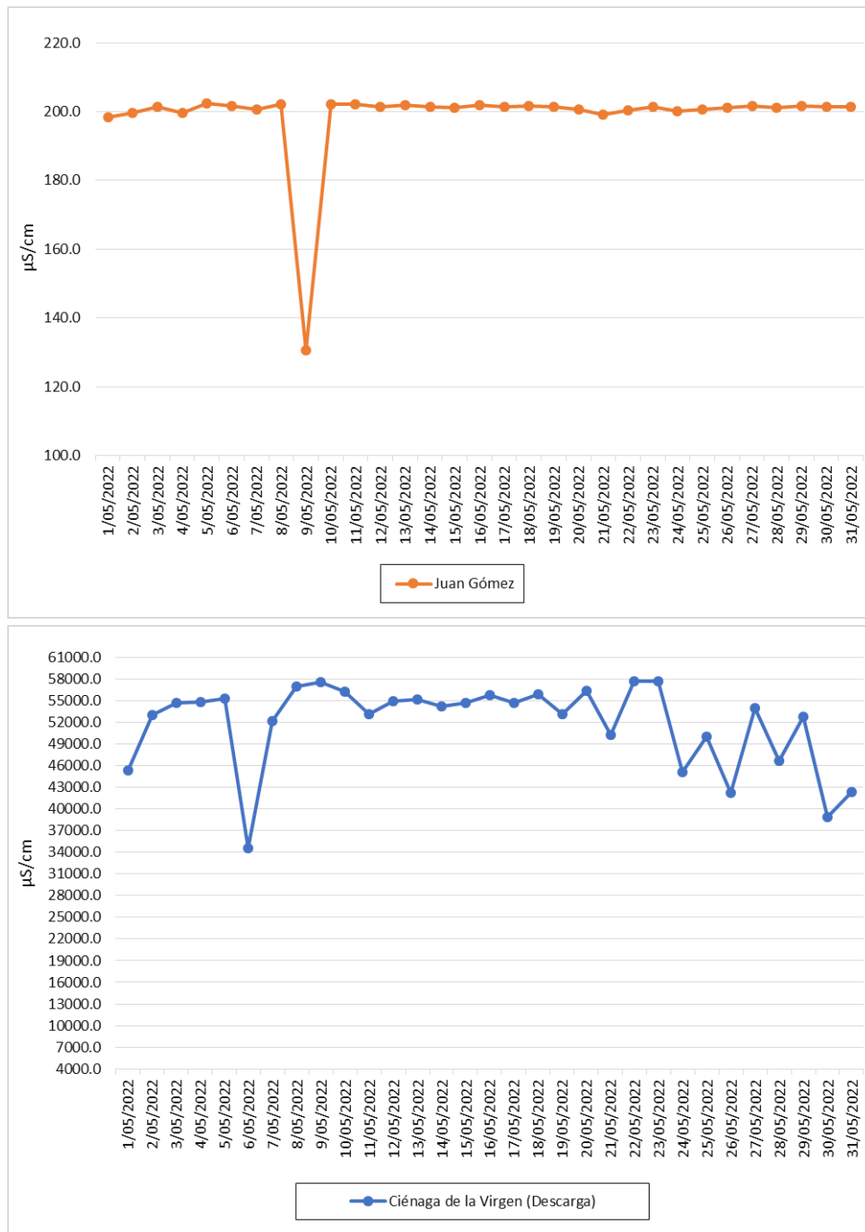
Ilustración 32 Conductividad del Agua Cálida Dulce
