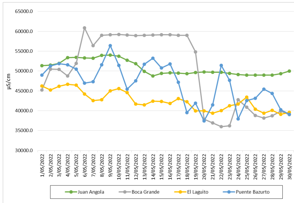
Ilustración 20 Conductividad del agua marina estuarina
