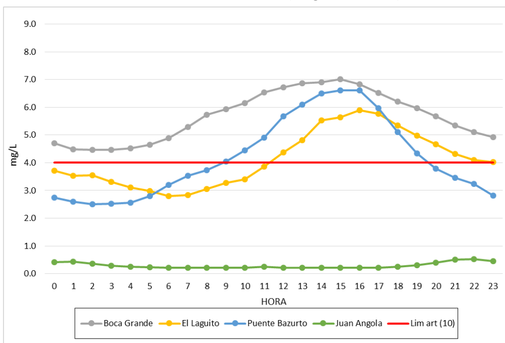
Ilustración 16 Perfil Horario (Oxígeno Disuelto)
