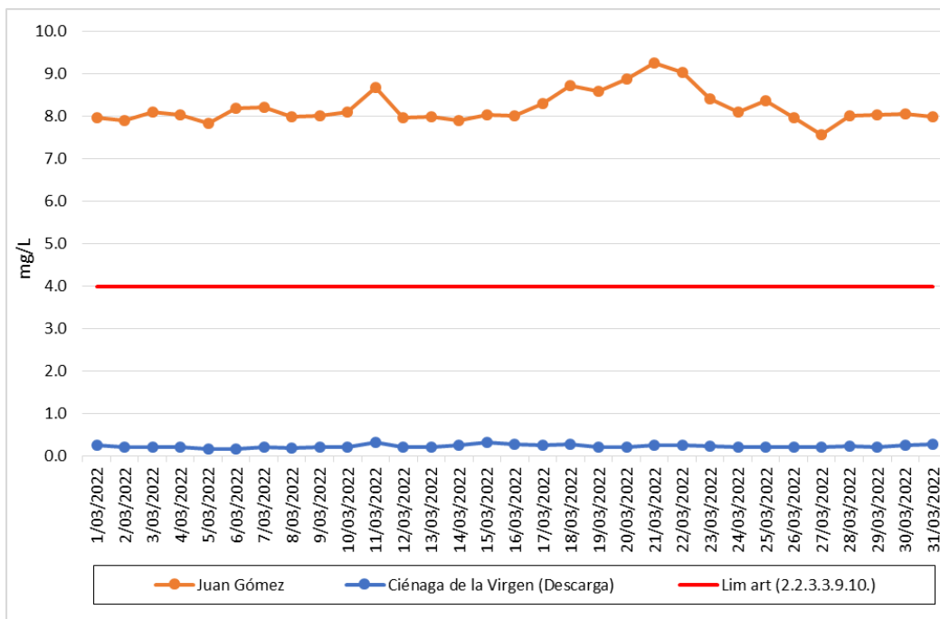
Ilustración 27 Oxígeno Disuelto del Agua Cálida Dulce
